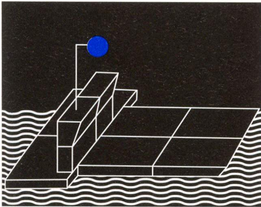
Artikel 3.14, lid 5: Bijkomende tekens van een duwstel dat door twee duwbotten naast elkaar wordt voortbewogen en dat gevaarlijke stoffen vervoert als 36a
