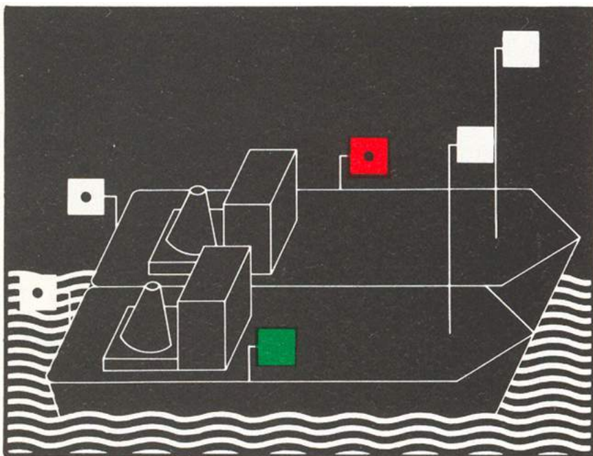
Artikel 3.11, lid 1: Gekoppeld samenstel; twee grote motorschepen.
